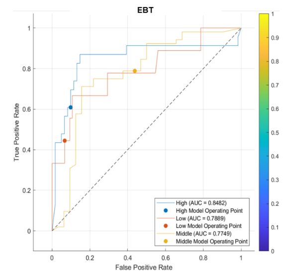
Fig. 5. AUC-ROC Curve of EBT.
