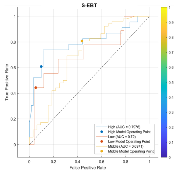
Fig. 7. AUC-ROC Curve of S-EBT.
