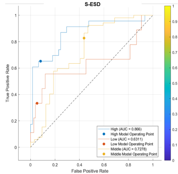
Fig. 6. AUC-ROC Curve of S-ESD.
