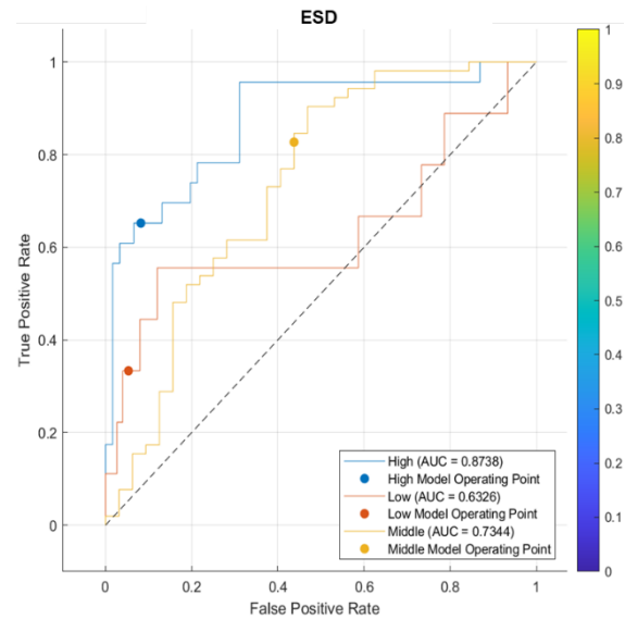
Fig. 3. AUC-ROC Curve of ESD.
